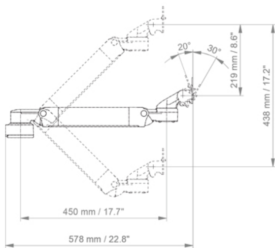
SIDE VIEW - VUE DE CÔTE - ZIJAAANZICHT
